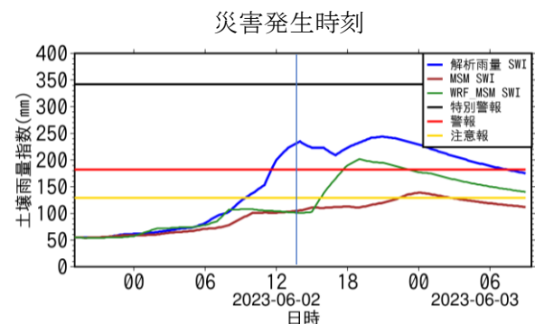
図-6 解析雨量、MSM、WRF の SWI
