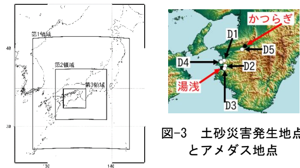
図-2 WRFの計算設定
